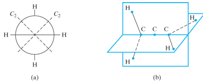
图 12.16: 联烯的两种视图。C=C=C 轴垂直于图 (a) 中纸张的平面。
